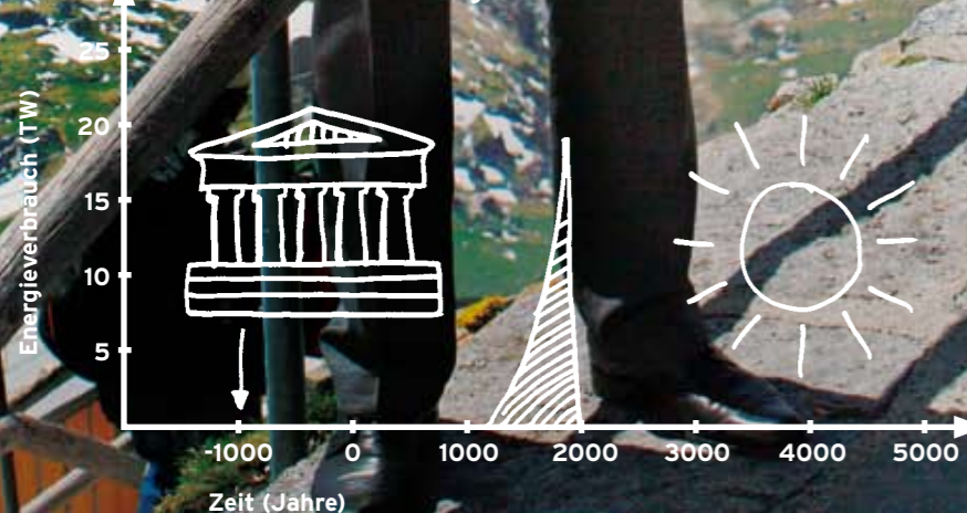
Fossiler Weltenergieverbrauch
